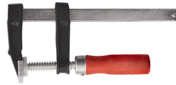
Размеры: 80*300 мм Тип: F-образная Материал: сталь
