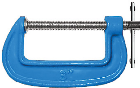
Размер: 75 мм Тип: G-образная Материал: сталь
